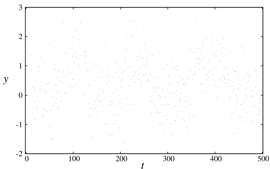
図 4: 観測値 y_t
