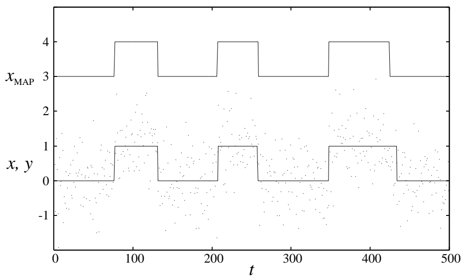
図 5: 下の実線: もとのデータ x_t , 上の実線: 事後確率を最大にする x_t の系列 x_{\text{MAP}}
